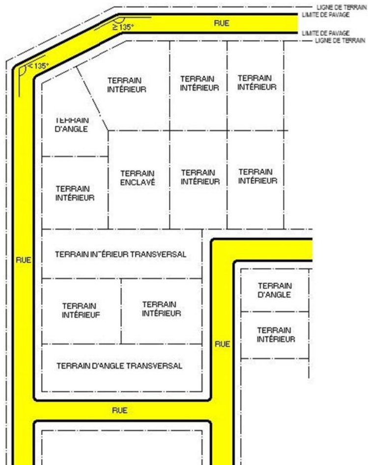
« illustration » : Dimensions d'un terrain
